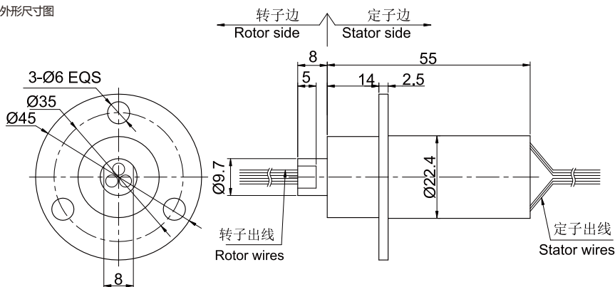
MW1630-IP65 外形尺寸图
