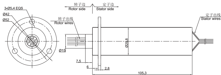
MW1181, MW1930, MW13605 外形尺寸图
